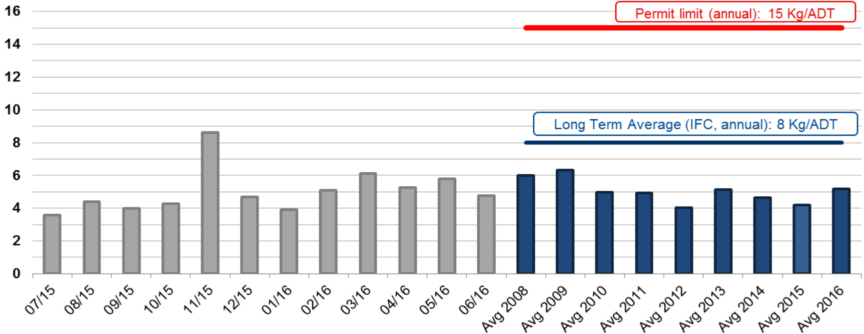
COD (DQO) - Kg/ADT
