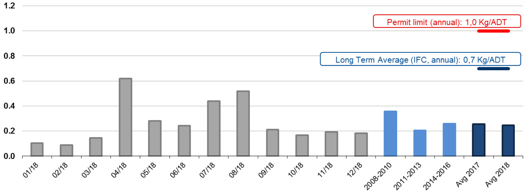
TSS (SST) - Kg/ADT
