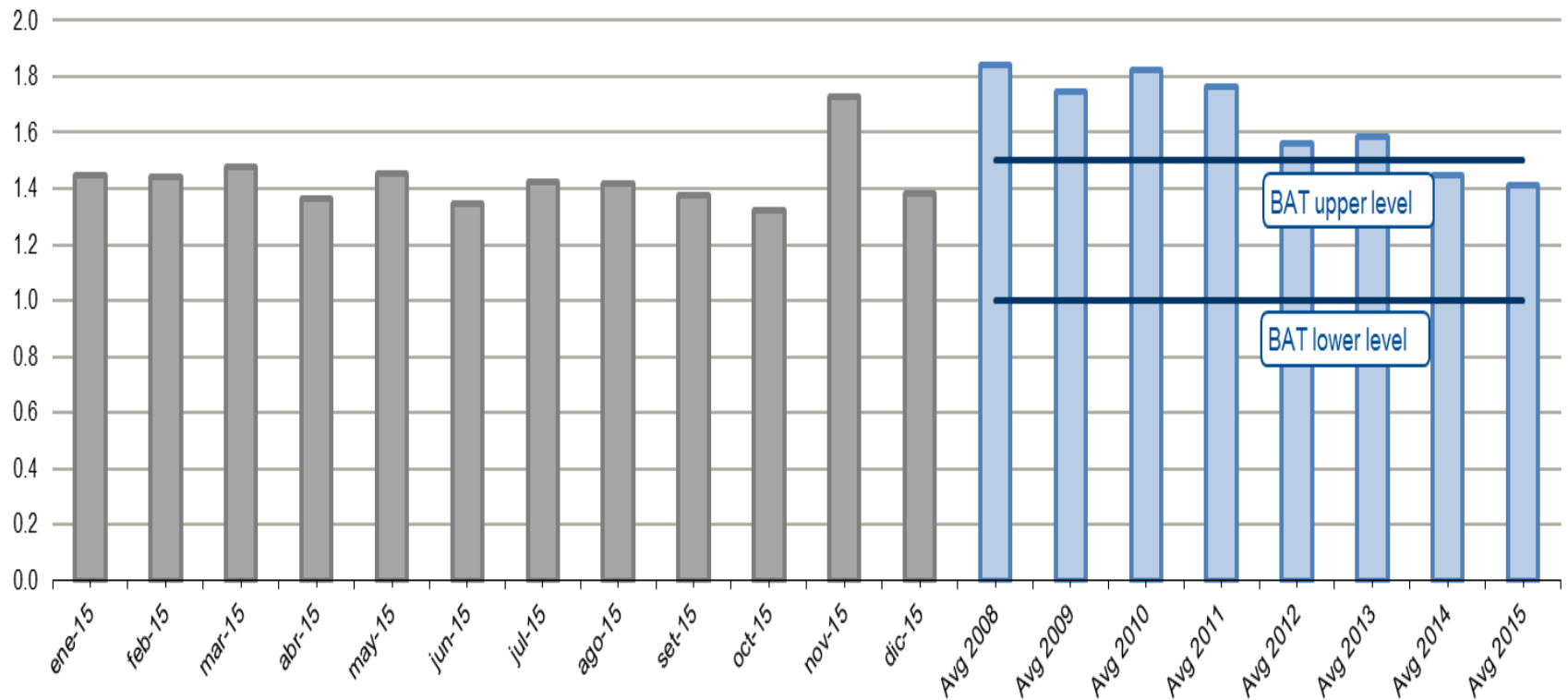
NOx - Kg/ADT
