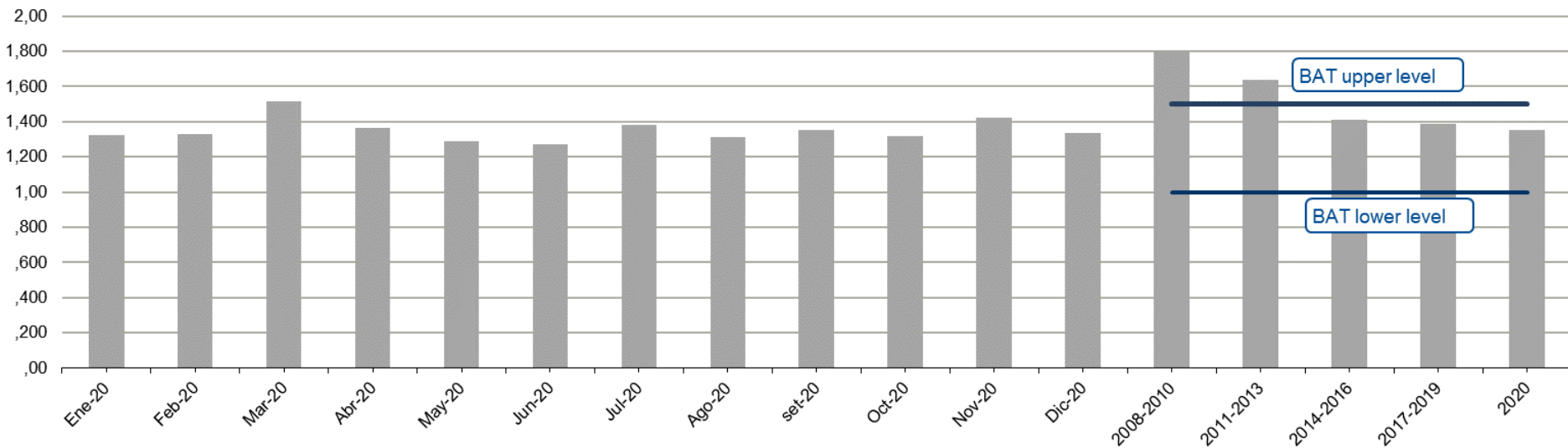
NOx - Kg/ADT
