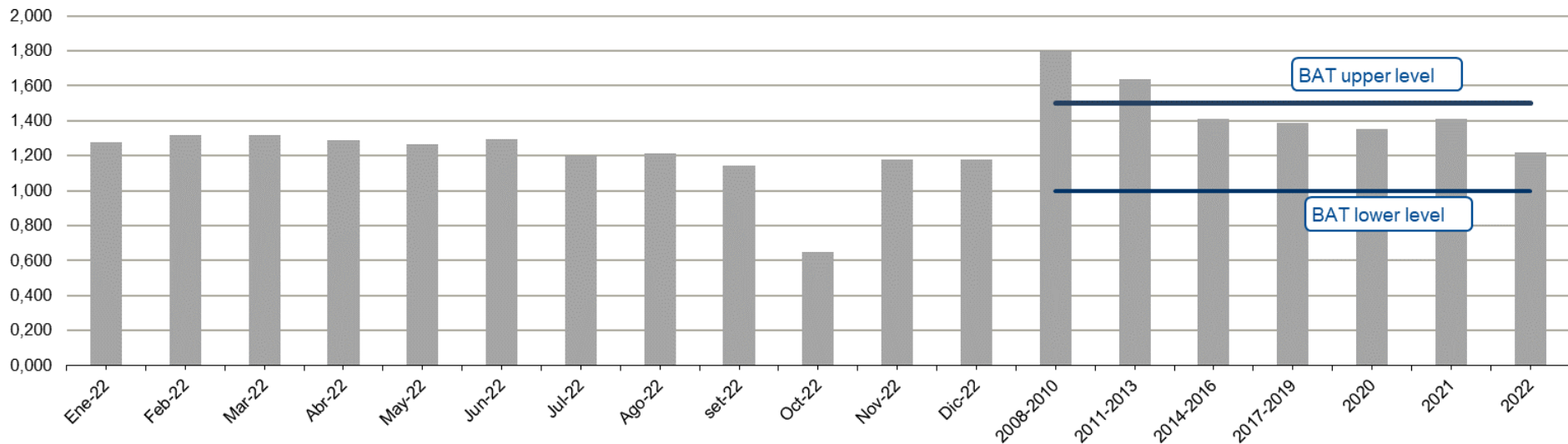
NOx - Kg/ADT
