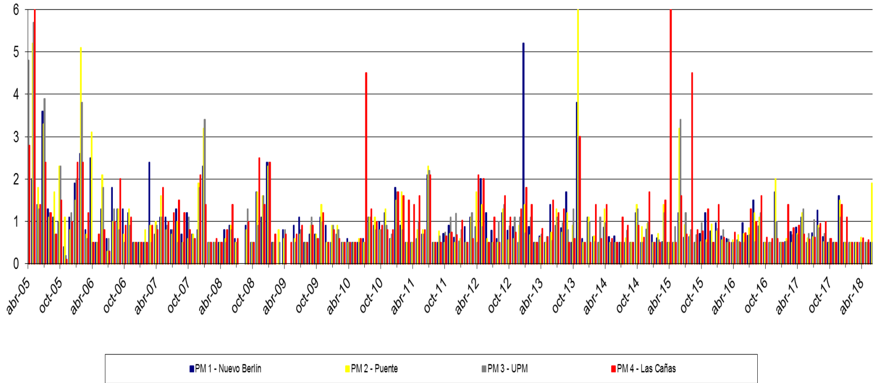
DBO - Concentración en el Río Uruguay (mg/L)
